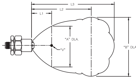
DE喷嘴喷雾形状尺寸
